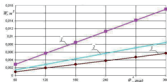
Рисунок 4 – Изменение транспортируемого объема снежной призмы для однозаходной, двухзаходной и трехзаходной фрез, где 1 – объем снежной призмы, вырезаемый однозаходной фрезой, м³; 2 – объем снежной призмы, вырезаемый одним заходом двухзаходной фрезы, м³; 3 – объем снежной призмы, вырезаемой одним заходом трехзаходной фрезы, м³
