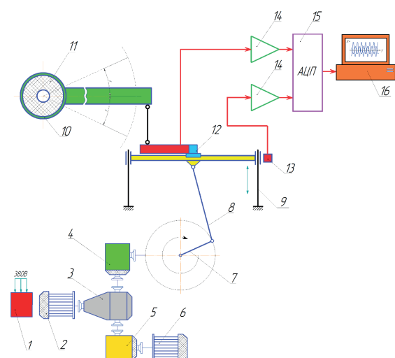
Рисунок 3 – Структурная схема модернизированного стенда. 1 – частотный преобразователь, 2 – электродвигатель, 3 – редуктор, 4 – коробка перемены передач ВА3-2109, 5 – мультипликатор, 6 – маховик, 7 – кривошип, 8 – шатун, 9 – направляющее устройство, 10 – рычаг подвески, 11 – испытуемый сайлентблок, 12 – датчик силы, 13 – датчик перемещения компьютер, 14 – усилитель, 15 – аналого-цифровой преобразователь, 16 – компьютер
