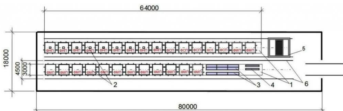
Рис. 1. Схема формовочного пролета стендовой линии «СЛ-7» с годовым выпуском ж/б изделий, позволяющим обеспечить строительство жилых домов общей площадью 30 000 м 2 .
